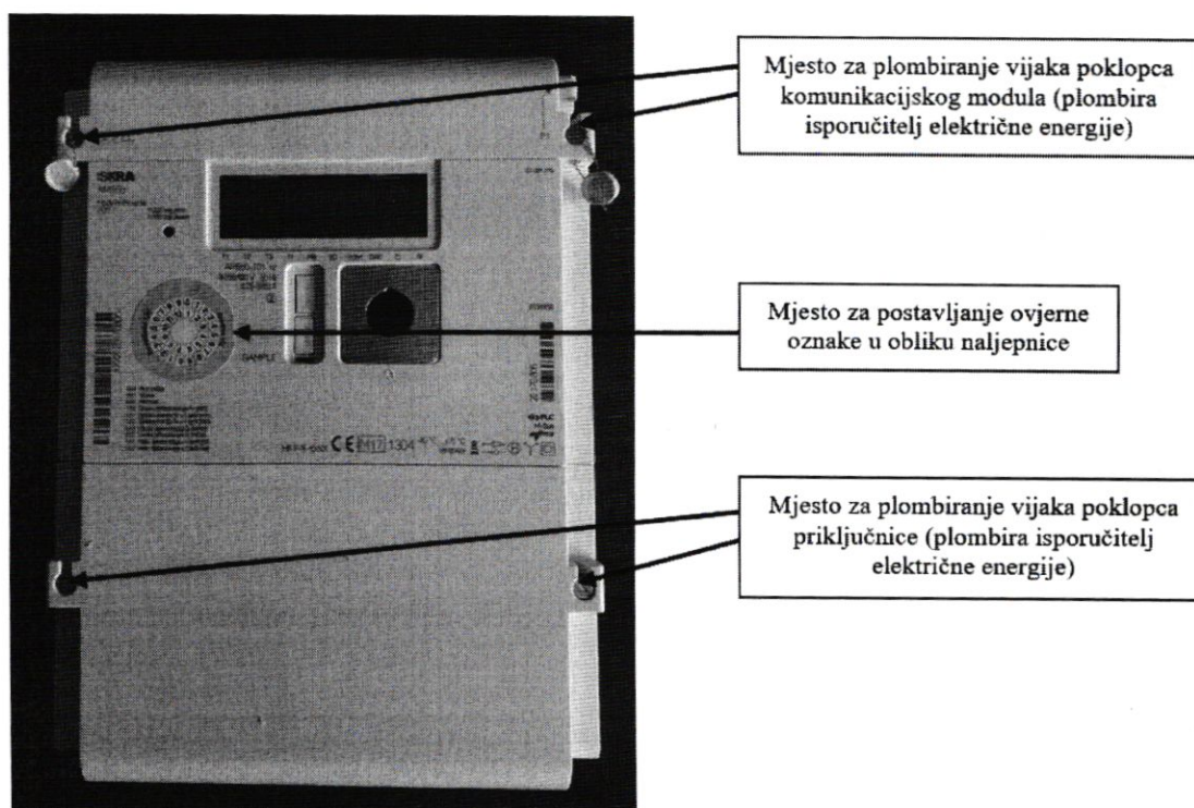
Slika 5. Slika brojila s označenim mjestima za ovjerne oznake i zaštitne plombe
